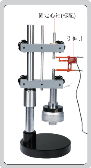
标定引伸计
